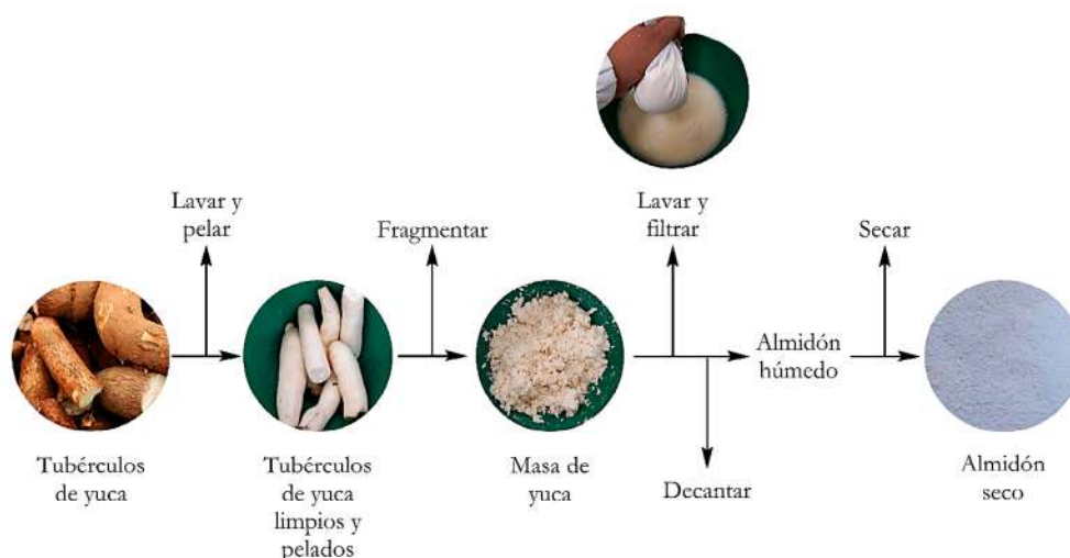
Figura 4. Diagrama de flujo para la extracción del almidón a partir de la yuca
