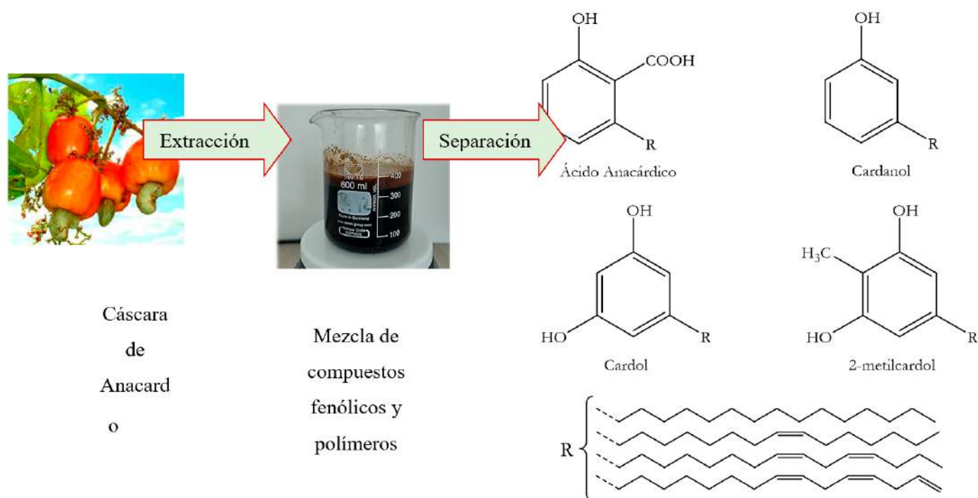
Figura 2. Estructura química de los compuestos del CNSL
